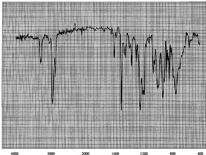
图1 炔螨特标样的红外光谱图
