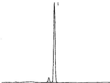
图 2 炔螨特原药高效液相色谱图
